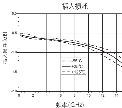
测试曲线(射频端口使用两根Φ25um长400um的键合线)
