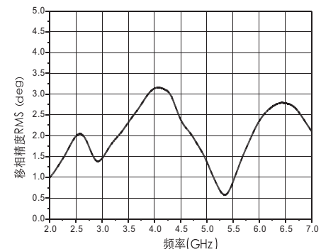
移相精度RMS
