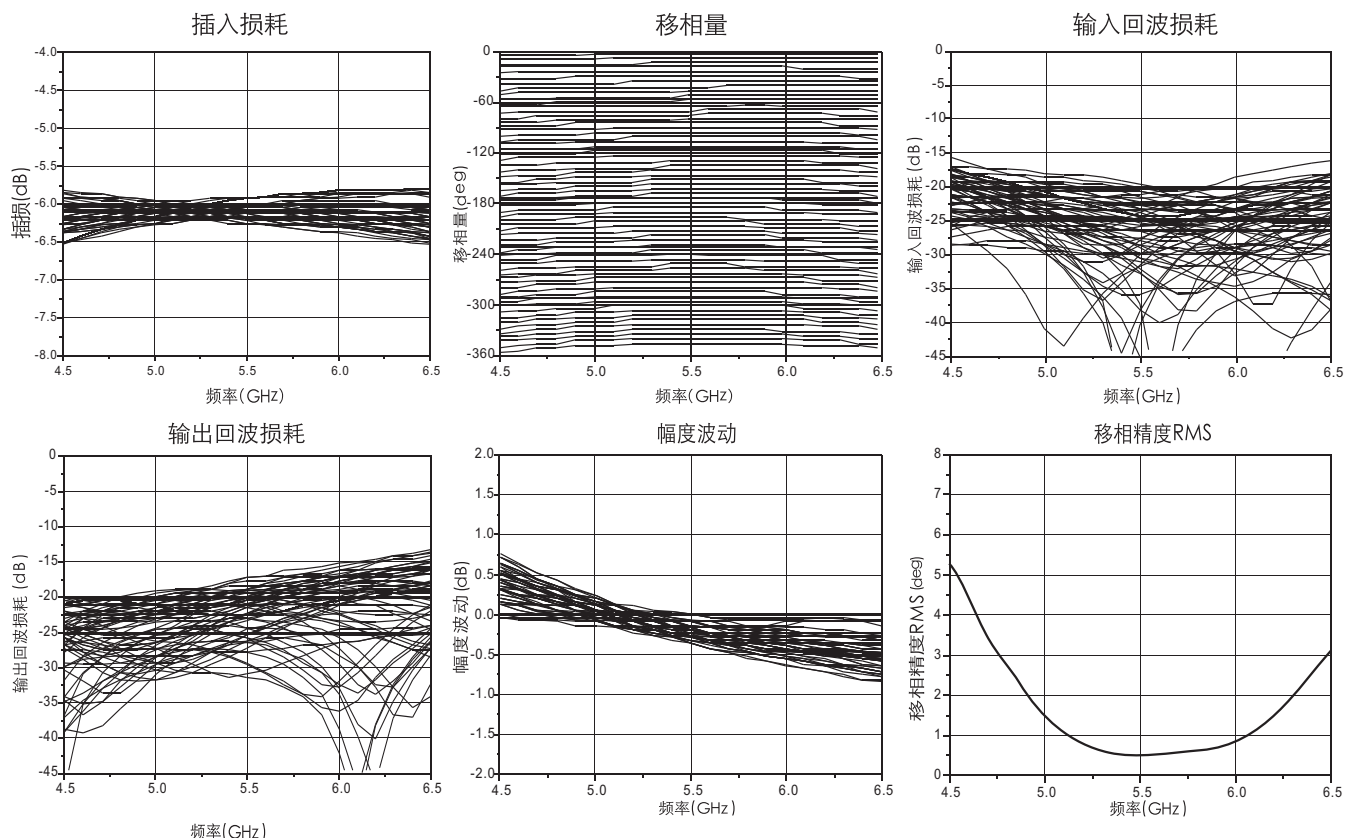
测试曲线(射频端口使用两根Φ25um长400um的键合线)
